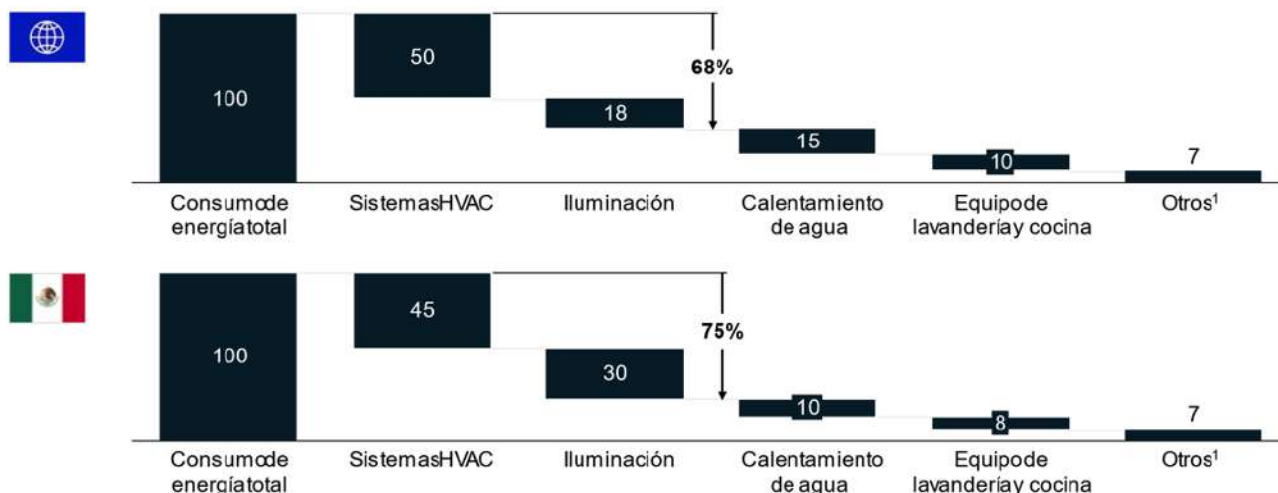
Distribución del consumo de energía en Hoteles, por fuente, %
